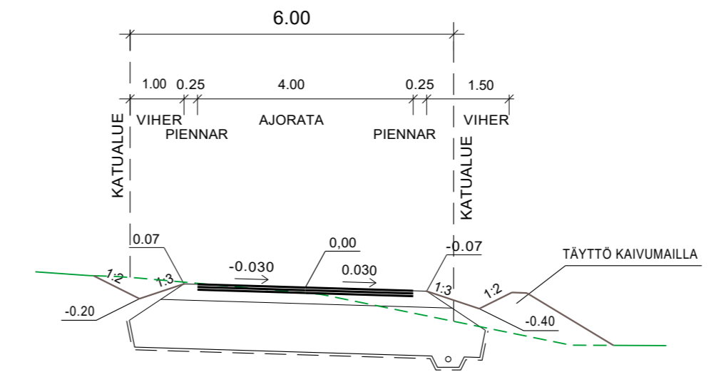
TYYPPIPOIKKILEIKKAUS PAALULTA 60 1:100
