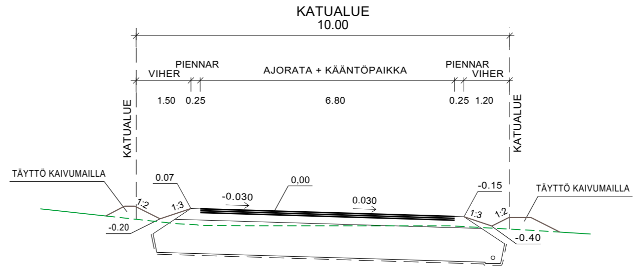
TYYPPIPOIKKILEIKKAUS PAALULTA 130 1:100
